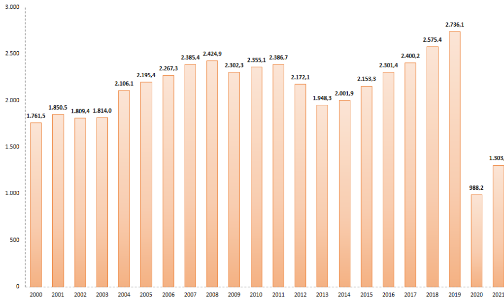
Figura 22. Evolución de los consumos finales de querosenos en la Comunidad de Madrid (ktep). Fuente: Exolum.
