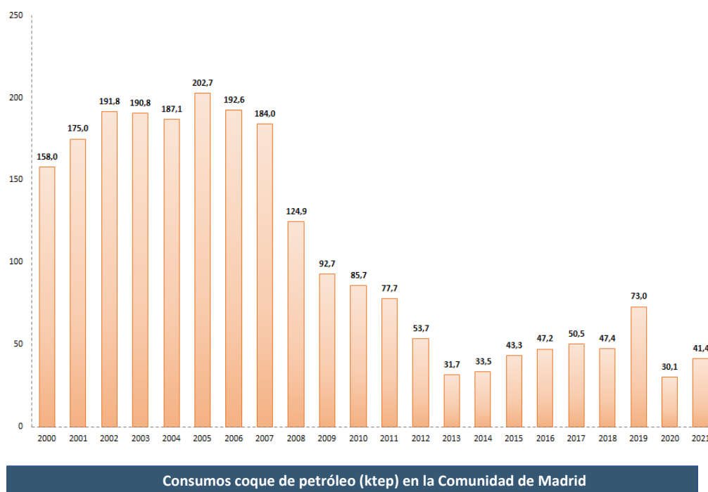
Figura 27 | Tabla 25. Evolución de los consumos finales de coque de petróleo en la Comunidad de Madrid (ktep). Fuente: Cementos Portland Valderribas.
