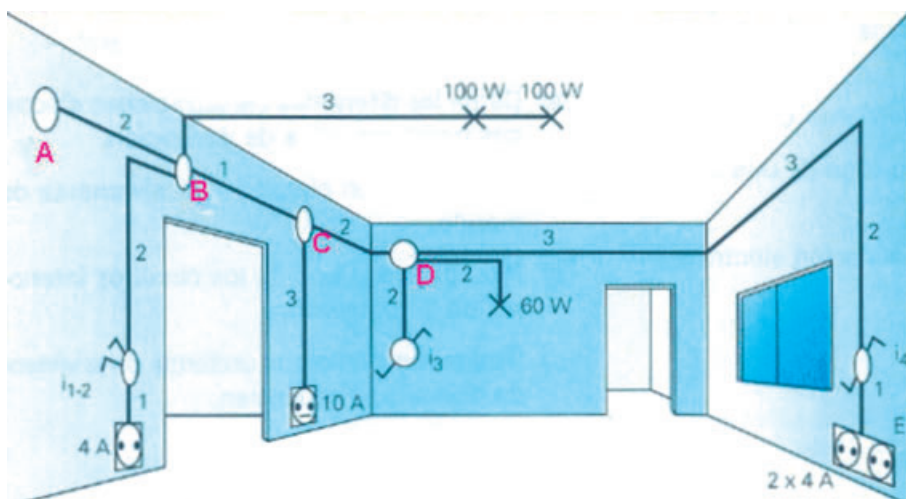
Figura 16. Instalación interior.
