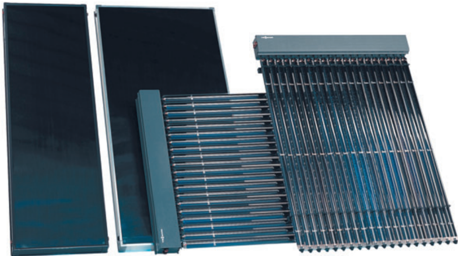
Figura 10. Ejemplos de tecnologías solares: Colectores solares Viessmann.
