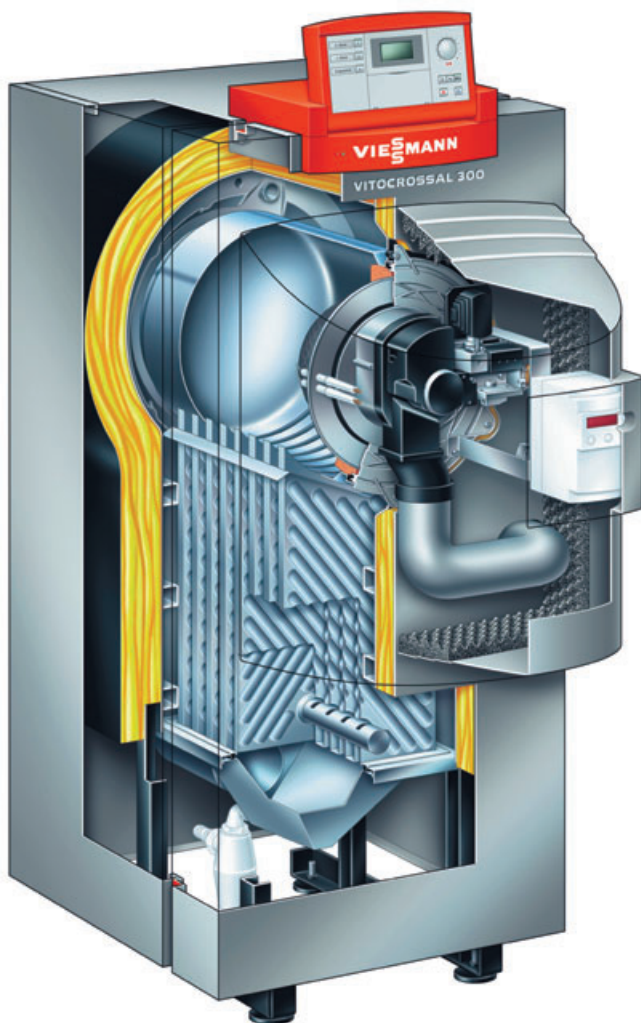
Figura 8. Vista seccionada de calderas de Condensación a gas de Viessmann, modelo Vitocrossal 300.
