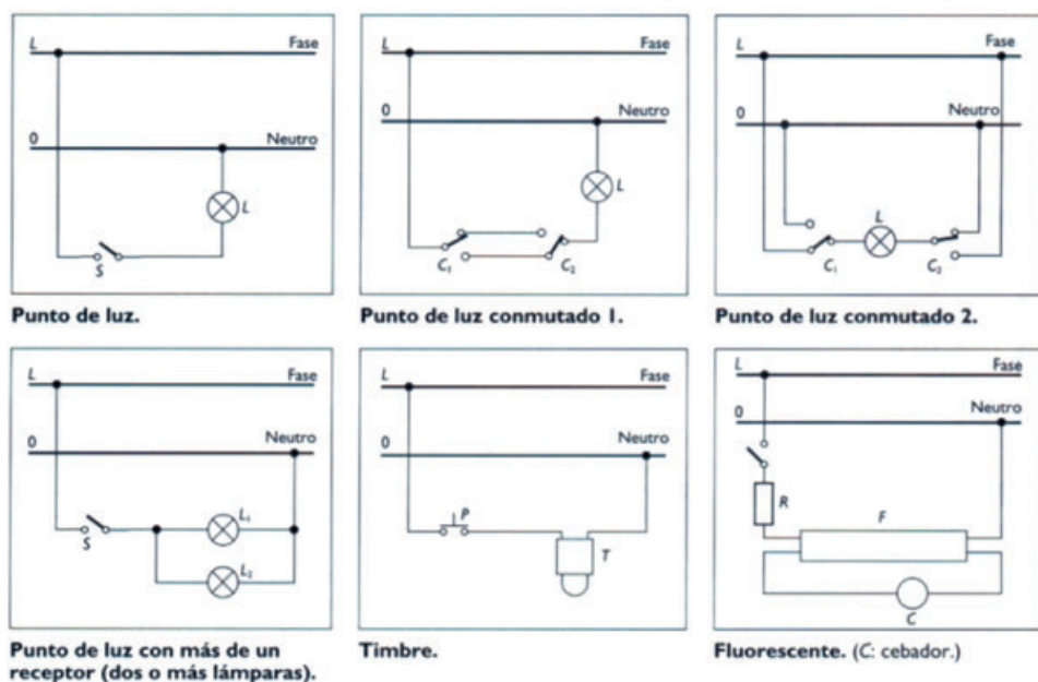
Figura 14. Esquemas de circuitos en vivienda.
