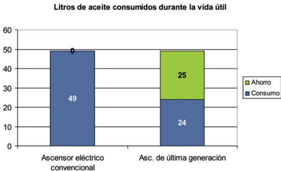
Figura 5. Consumo de aceite comparado con ascensores eléctricos.
