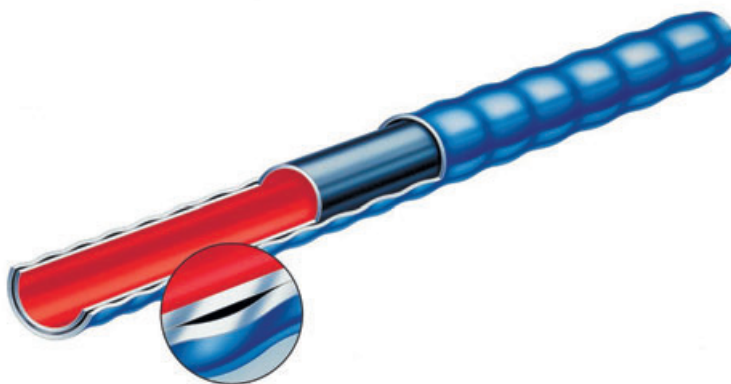
Figura 3. Tubo Duplex de la Vitomax 300.
