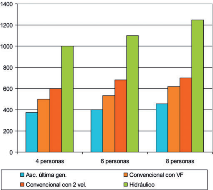
Figura 1. Consumos en kWh.
