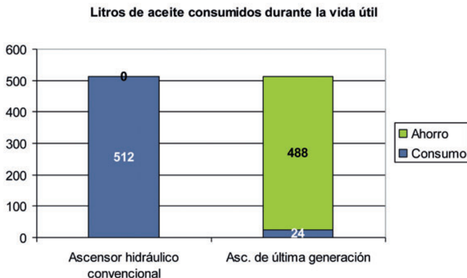
Figura 4. Consumo de aceite comparado con ascensores hidráulicos.
