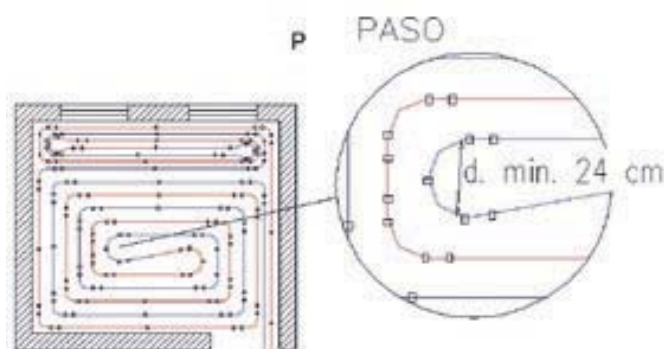
Figura 3.1b. Detalle circuito
