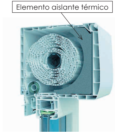
Foto 6.2. Cajón Protex. Valor Transmitancia térmica U=0,82 \text{ W/m}^2\text{K} . Deceuninck.
