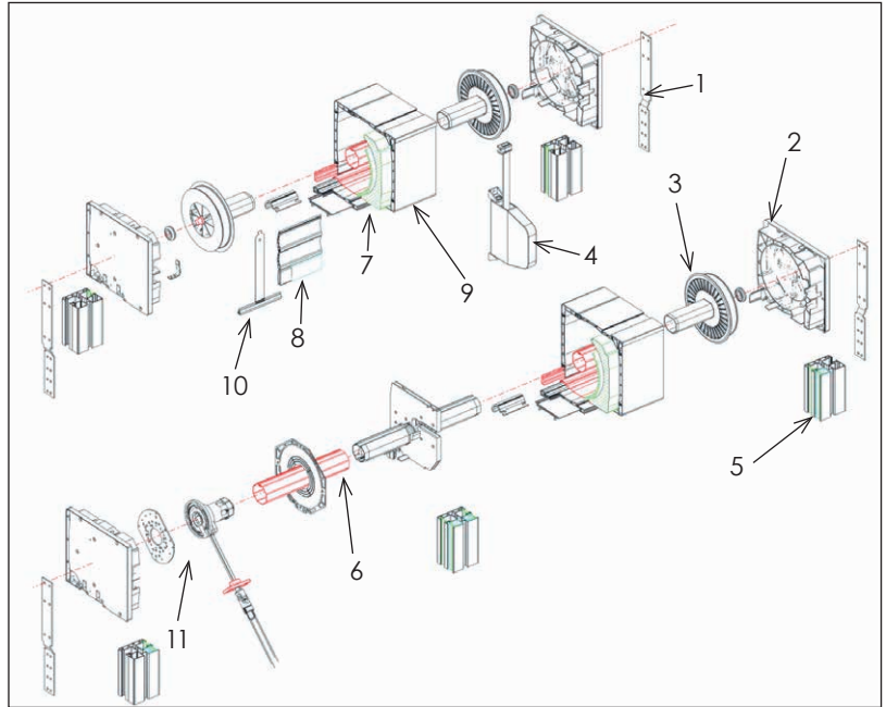
Foto 6.1. Componentes cajón Protex de Deceuninck
