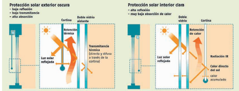
Figura 9.6. Impacto de la posición y color de las protecciones solares en las ganancias de calor.
