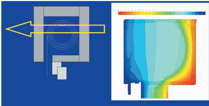
Foto 6.1. Flujo de calor cajón Protex de Deceuninck.
