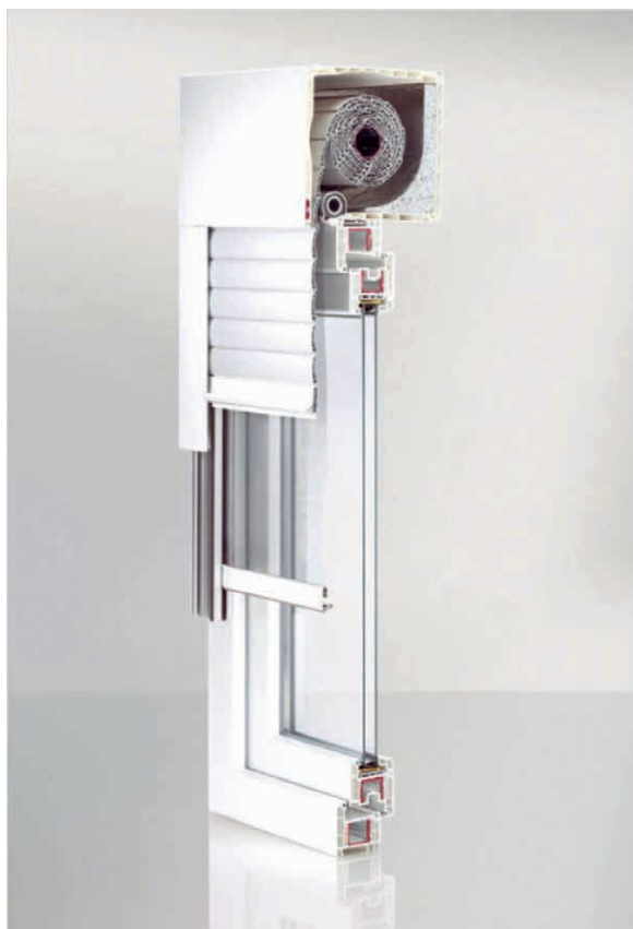
Foto 12.1. Sistema de 70 mm con cajón de persiana de alta Eficiencia. Fuente: REHAU.
