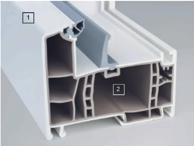
Foto 12.3. Detalle del sistema GENEEO® fabricado mediante la coextrusión de dos polimeros (RAU PVC y RAU FIPRO®).
