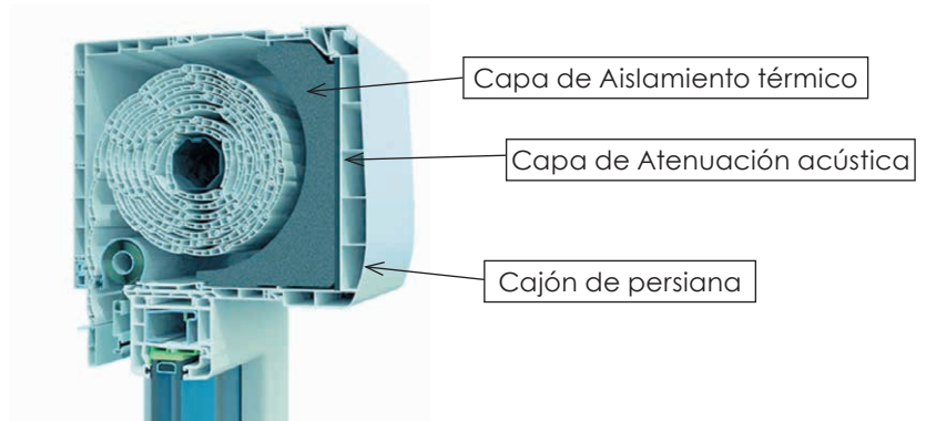
Foto 6.3. Cajón Protex. Atenuación Acústica 42 (-1;-3) dB. Deceuninck
