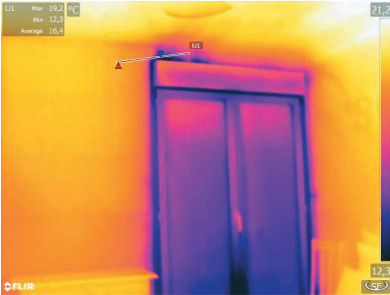
Foto 11.23. Capialzado con entradas de aire en la parte superior
