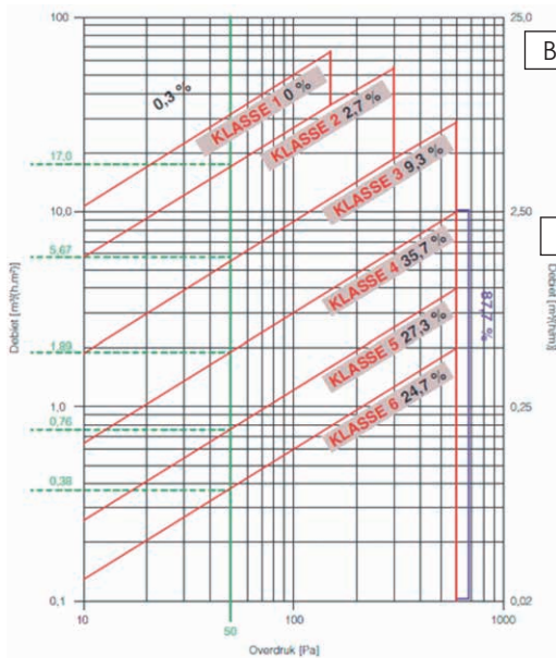
Figura 8.10. Resultados de bandas pre-comprimidas según EN 12207.
