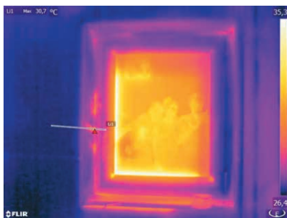
Fotos 11.3 y 11.4. Vivienda pasiva en ejecución en Rivas Vaciamadrid. Las exigencias de estanqueidad son máximas para este tipo de viviendas que no deben superar el valor n50 de 0,6 \text{ren/h} .
