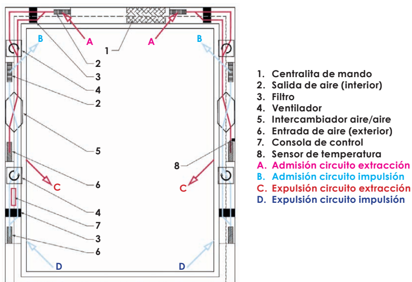
Figura 12.4. Esquema de funcionamiento del sistema GENE O INOVENT®.
