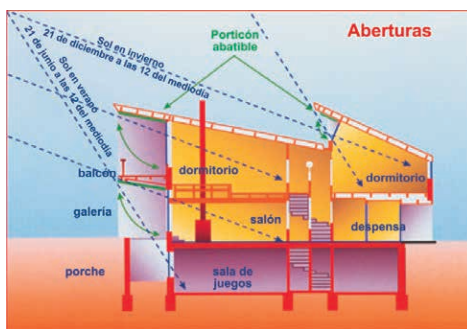
Figura 9.1. El estudio de una sección transversal de los huecos de un edificio permite determinar los niveles y el calendario de la luz del día y el aporte solar.
