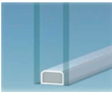
Foto 13.3. Doble acristalamiento tradicional sGG CLIMALIT 4/6/4 básico. Fuente: Saint-Gobain Glass
