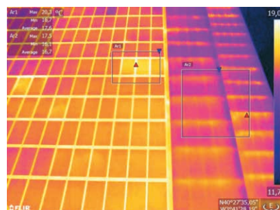
Foto 11.29 y 11.30. Se detectan dos vidrios (Ar1) con mayor transmisión de calor. Tratándose de una zona diáfana en el interior, debemos ya de continuar la inspección desde el interior para detectar el motivo de esta diferencia de temperatura.
