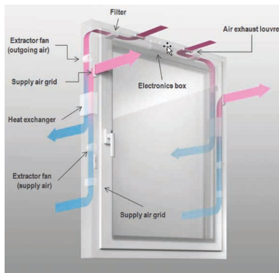
Figura 12.3. Esquema de funcionamiento del revolucionario sistema GENE O INOVENT®.
