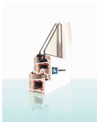
Foto 13.4. Carpintería muy aislante realizada en PVC con doble acristalamiento. Fuente: Kömmerling.
