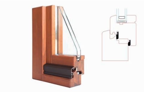
Foto 4.3. Ventana DJ68 CARINBISA.
