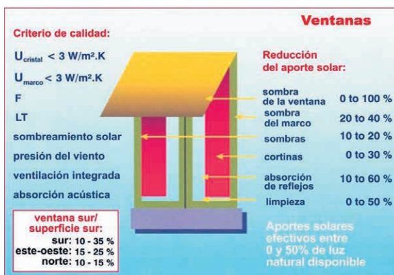
Figura 9.2. Lista de criterios que intervienen en el rendimiento térmico de las ventanas.
