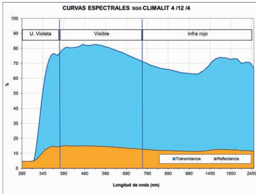
Gráfico 2.6. Comportamiento de un acristalamiento incoloro sin protección solar y no selectivo.
