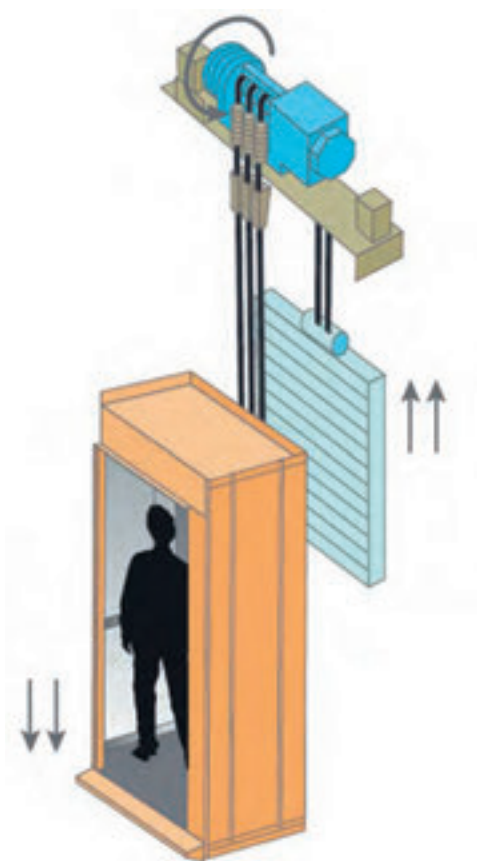
Figura 2. Cuando el ascensor baja cargado o sube vacío, el motor genera energía. Fuente: OTIS.
