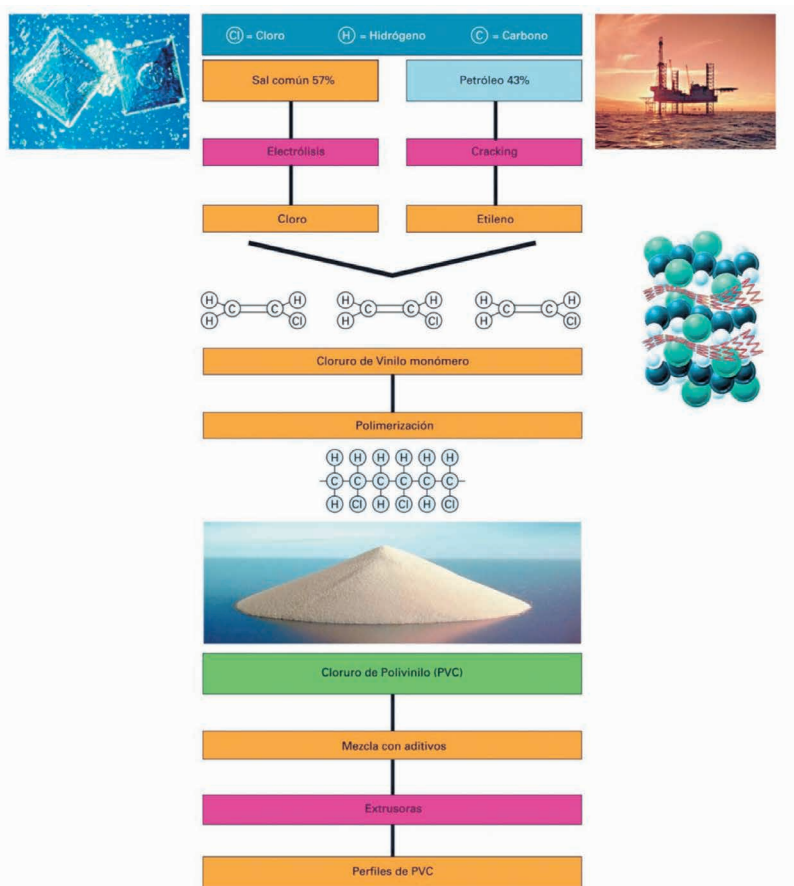
Figura 3.1. Proceso productivo de los perfiles de PVC.
