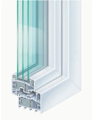
Figura 3.2. Sistema 88plus Passivhaus (KÖMMERLING).
