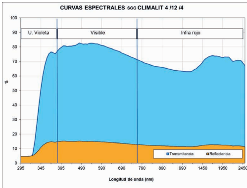
Gráfico 2.6. Comportamiento de un acristalamiento incoloro sin protección solar y no selectivo.
