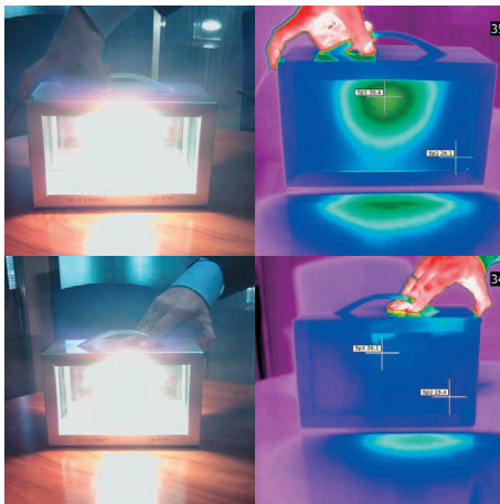
Foto 2.7. Arriba doble acristalamiento tradicional. Abajo sGG CLIMALIT PLUS (Doble acristalamiento ATR). Fuente: sGG CLIMALIT– Saint-Gobain Glass.
