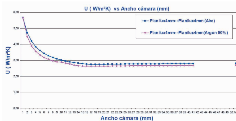
Gráfico 2.1. Evolución de la reducción de U con el espesor de la cámara y presencia de gas.
