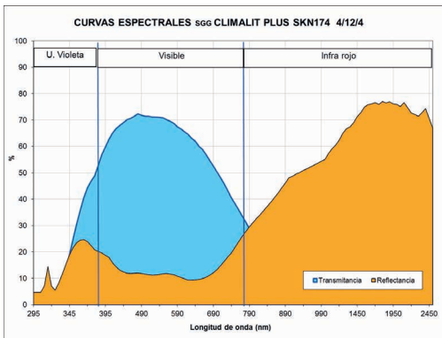
Gráfico 2.7. Comportamiento de un acristalamiento altamente selectivo.
