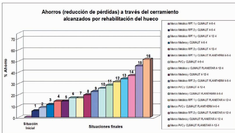
Gráfico 2.5. Comparativa de ahorros (disminución de U) a través de la ventana por cambio de doble acristalamiento a doble acristalamiento ATR. Fuente: SGG CLIMALIT– Saint-Gobain Glass.
