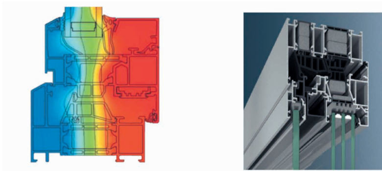
Figura 5.4. Líneas de Temperatura. Sistema con U_f=0,85
