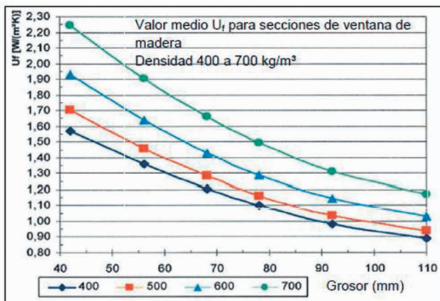
Gráfico 4.1. Transmitancia térmica de marcos de madera.
