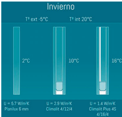
Figura 2.2. Simulación de temperaturas interiores de un acristalamiento en función de su valor U. Fuente: sgc CLIMALIT– Saint-Gobain Glass.
