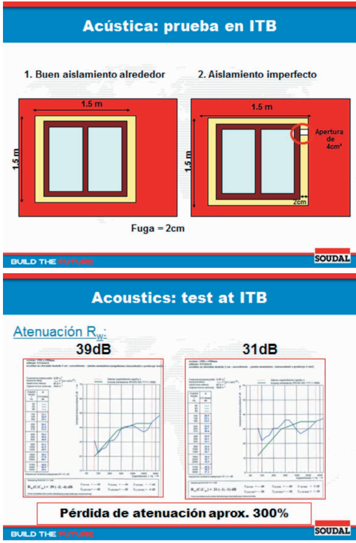
Figura 8.11. Resultado de ensayos ITB. Fuente: SOUDAL.
