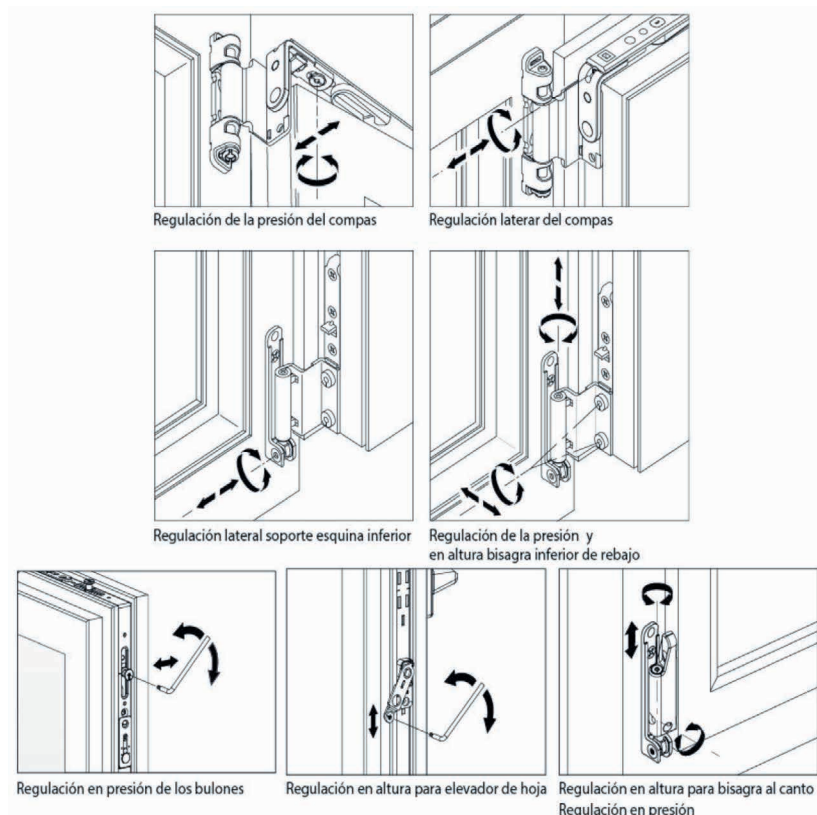
Figura 7.10. Regulación de herraje oscilobatiente
