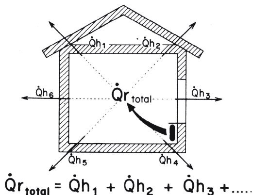
Figura 2.2. Potencia calorífica.
