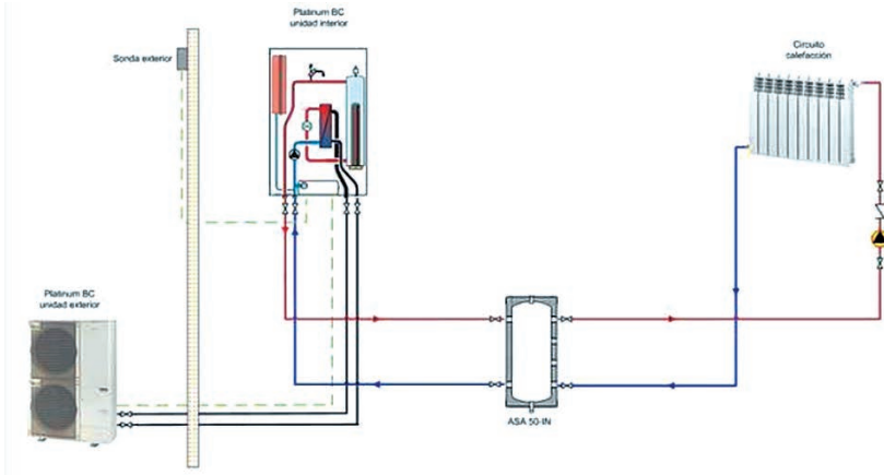
Figura 4.6. Esquema hidráulico de una instalación de bomba de calor con radiadores.
