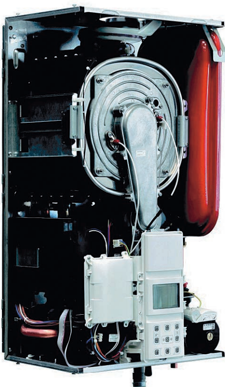
Foto 3.1. Interior de una caldera de condensación.
