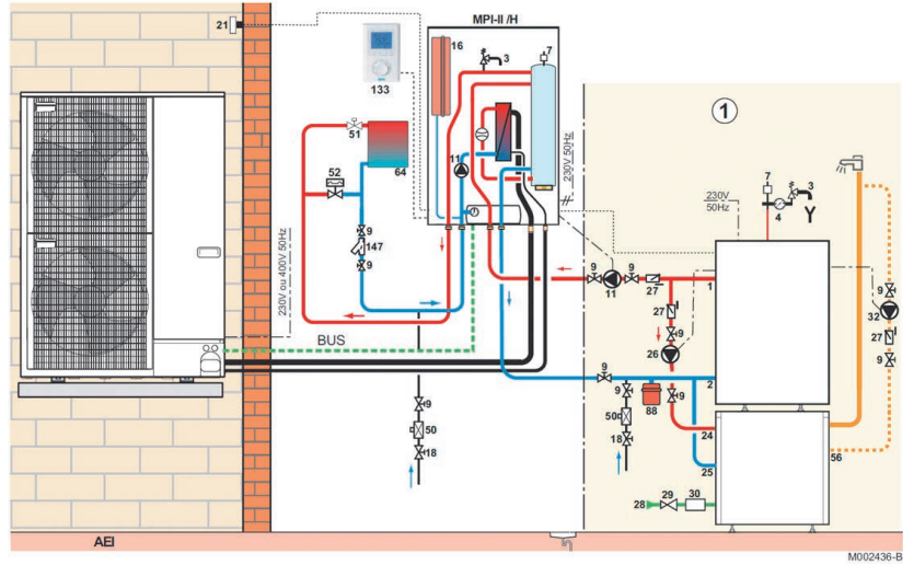
Figura 4.13. Esquema de instalación de generador de calor + bomba de calor.
