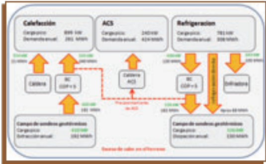
Figura 4. Concepto energético con datos energéticos Nota: BC = bomba de calor
