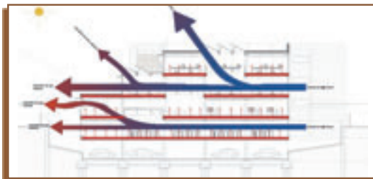
Esquema del sistema de refrigeración pasiva mediante la interacción de la ventilación y la inercia
