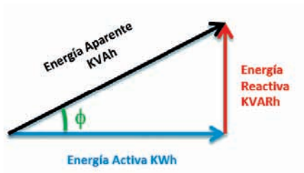
Figura 3. Triángulo de potencias.
