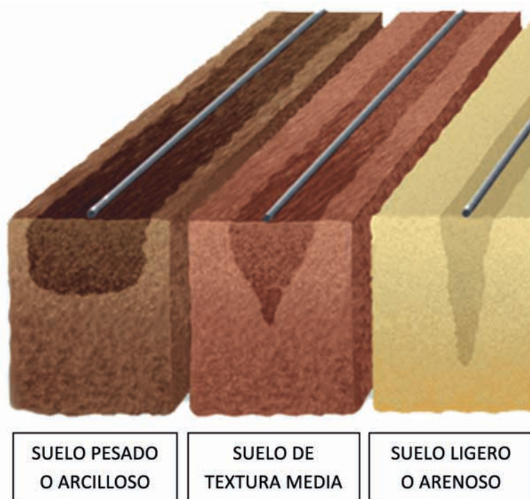
Figura 3. Comportamiento del bulbo húmedo según la textura del suelo. Fuente: Regaber
