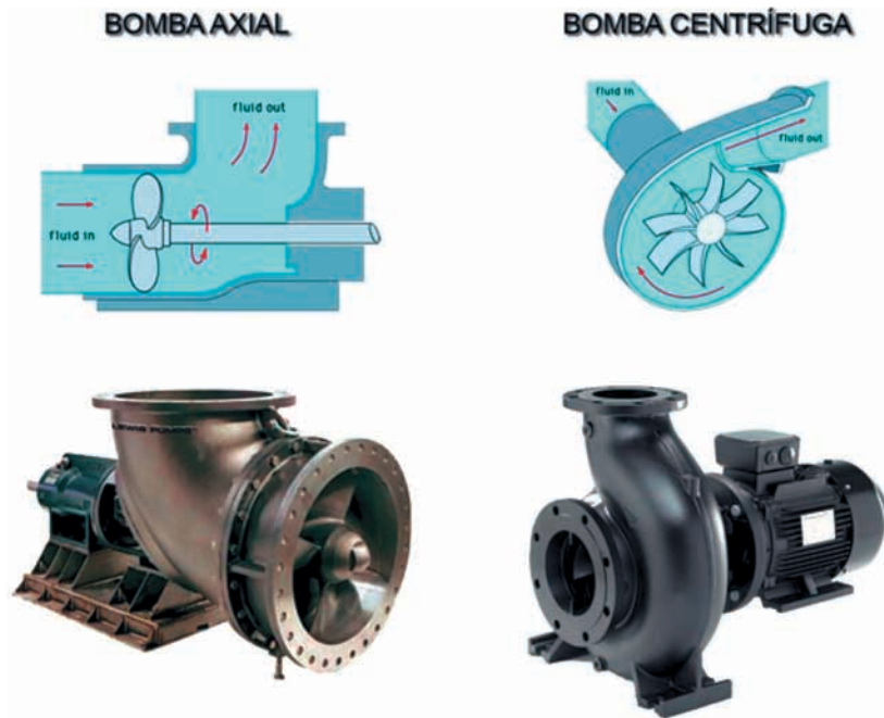
Figura 1. Tipos de bombas. Fuente: Audit Irrigation
