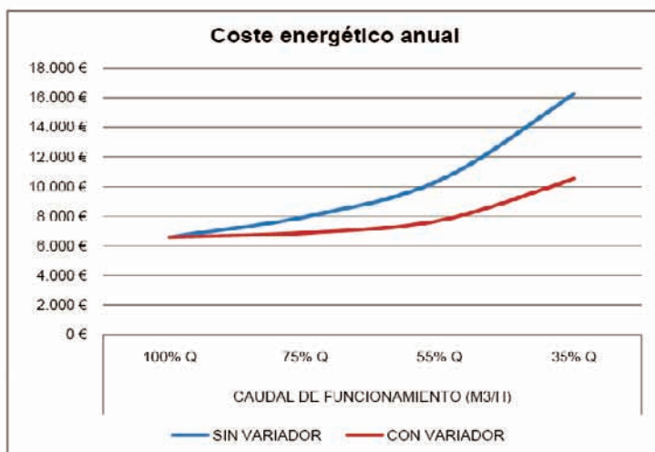
Gráfico 6. Simulaciones de riego y consumos energéticos. Fuente: Audit Irrigation
