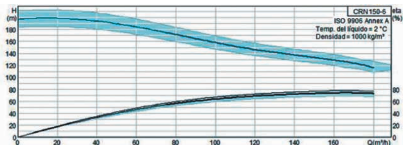
Gráfico 2. Curva característica de una bomba con sus tolerancias. Fuente: Wincaps de Grundfos
