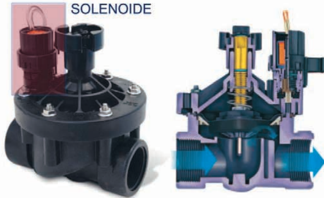
Figura 1. Electroválvula y solenoide. Fuente: Rainbird
