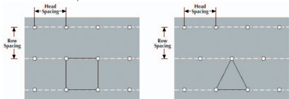
Figura 1. Distancias en marco cuadrado y triangular. Fuente: Hunter Industries
