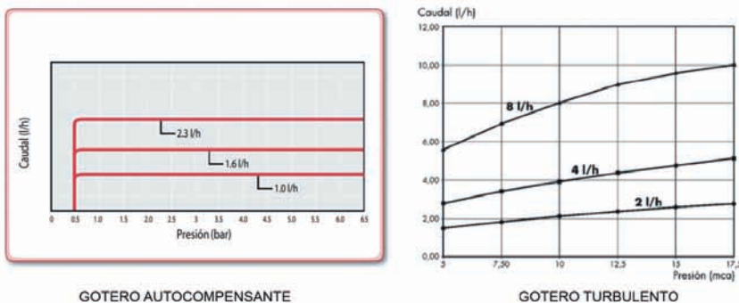
Gráfico 4. Comparativa gotero autocompensante gotero turbulento. Fuente: Regaber
