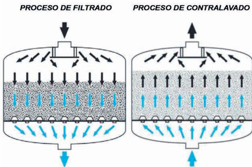
Figura 2. Detalle de procesos de filtrado y contralavado de un filtro de arena. Fuente: Regaber
