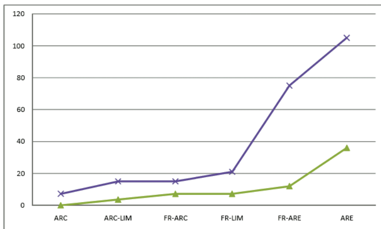
Gráfico 2. Velocidades de Infiltración en función de la textura del suelo. Fuente: Audit Irrigation
