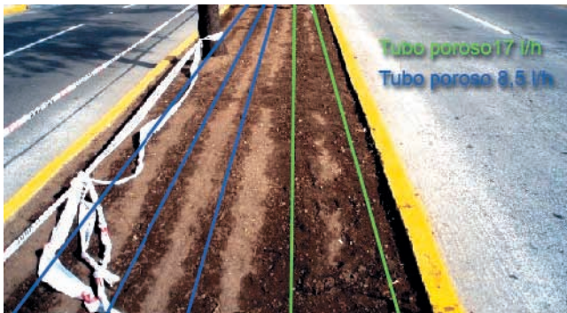
Figura 10. Distribución de riego no uniforme por empleo de goteros de distinto caudal. Fuente: Audit Irrigation
