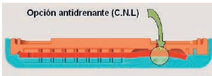
Figura 5. Detalle de un gotero de pastilla antidrenante. Fuente: Regaber
