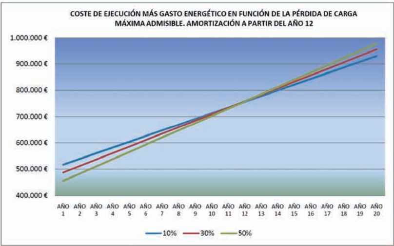
Gráfico 2. Amortización de la instalación. Fuente: Audit Irrigation
