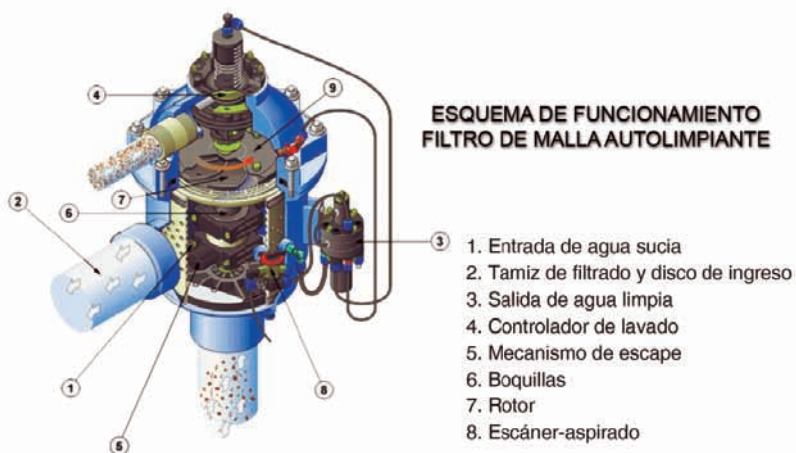
Figura 5. Esquema de funcionamiento de filtro de malla autolimpiante. Fuente: Regaber
