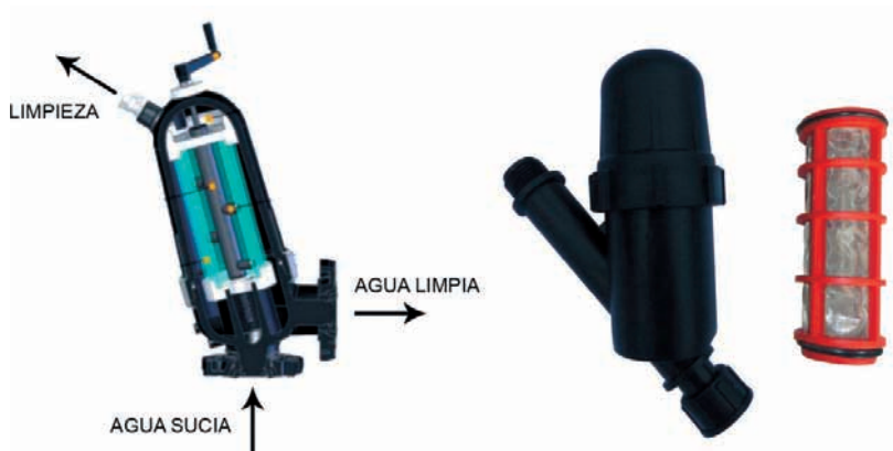
Figura 3. Sistema de filtración de filtro de malla. Fuente: Varios
