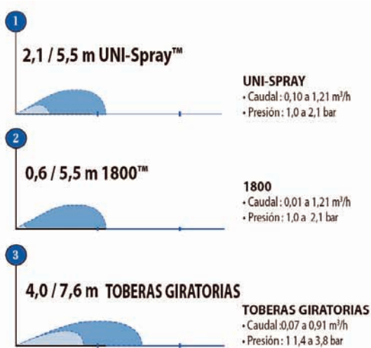
Figura 5. Alcances, caudales y presiones de una serie de difusores. Fuente: Rainbird
