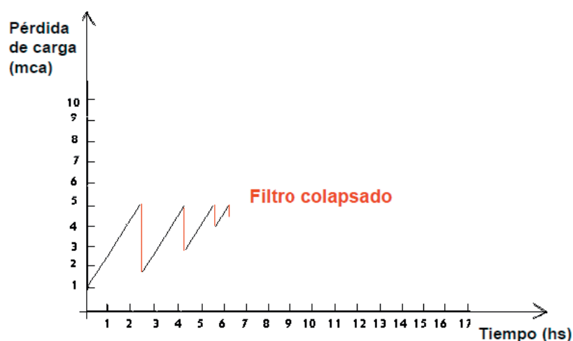
Figura 5. Gráfica de un contralavado incorrecto de un filtro autolimpiante. Fuente: Regaber
