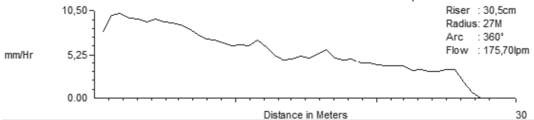
Gráfico 4. Perfil de un aspersor. Fuente: Programa SpacePro™ del C.I.T.
