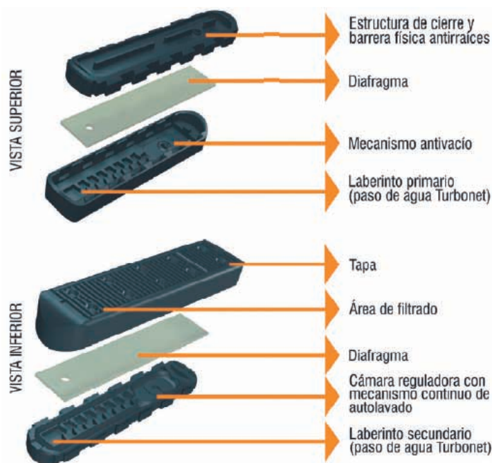
Figura 6. Partes de un gotero autocompensante con sistema antiraíces. Fuente: Regaber
