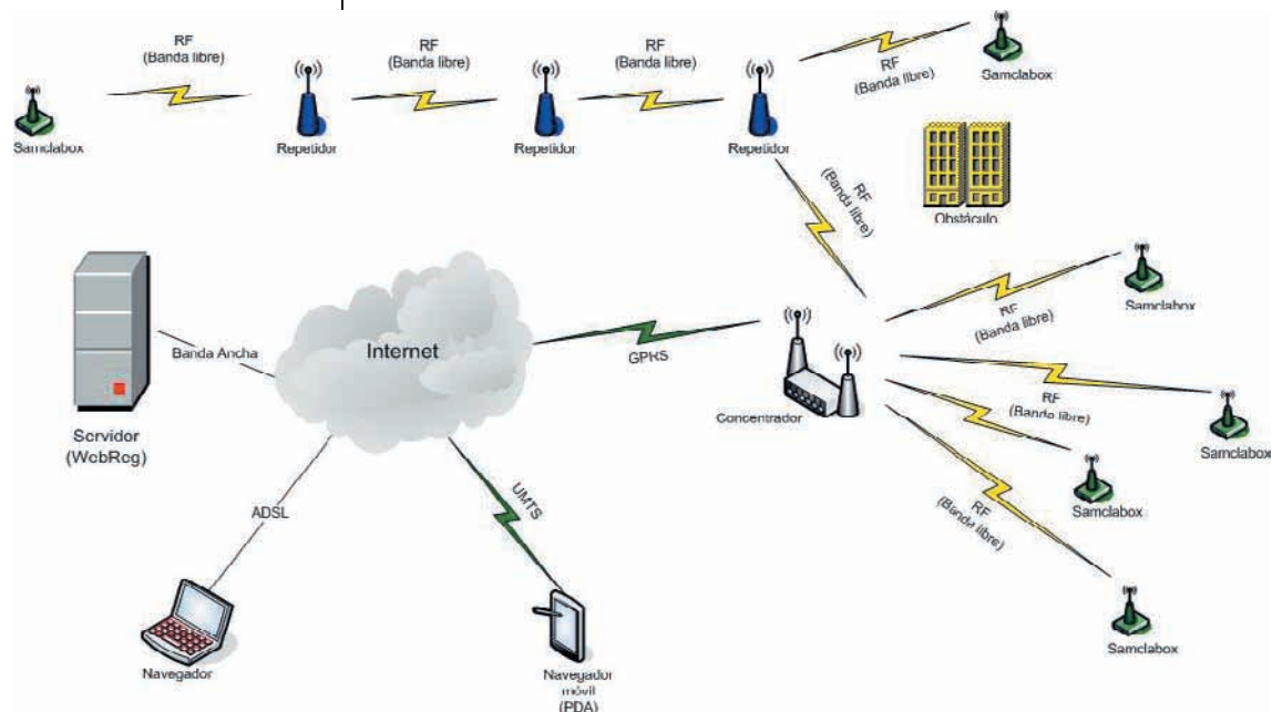
Figura 1. Esquema de comunicaciones. Fuente: Samclab
