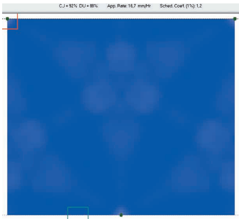
Figura 2. Densograma. Fuente:Programa SpacePro™ del C.I.T.
