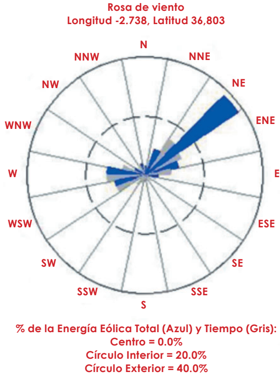
Figura 6. Rosa de viento. Fuente: Electri.
