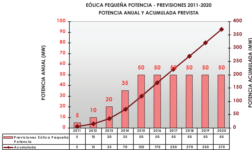
Figura 1. Eólica pequeña potencia. Previsiones de desarrollo en España, horizonte 2020. Fuente: IDAE.
