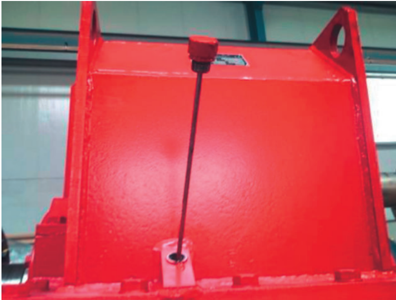
Figura 6. Varilla de comprobación de nivel de aceite de la multiplicadora. Verificación del nivel de aceite. Fuente: Electrica Wind, S.L.
