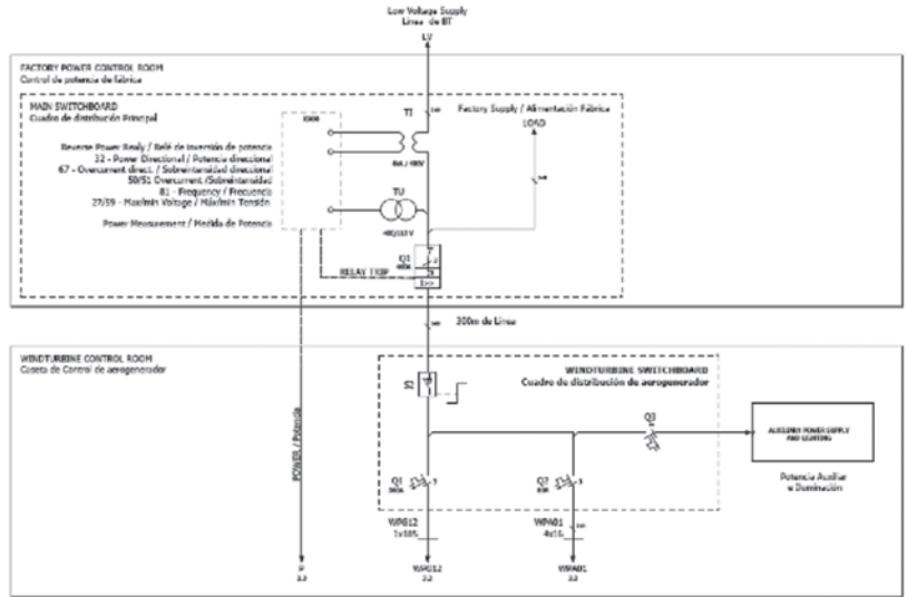
Figura 9. Esquema unifilar. Fuente: Electricia.
