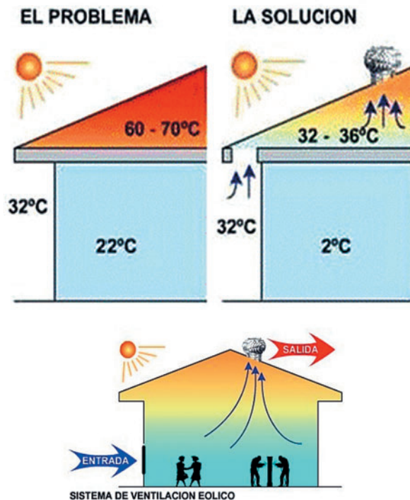
Figura 3. Sistema de ventilación con el extractor eólico. Fuente: Ilustración de EXTRACTORES EÓLICOS ATLANTIS
