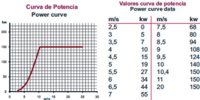
Figura 7. Curva de potencia Garbí 150/28. Fuente: Electri.
