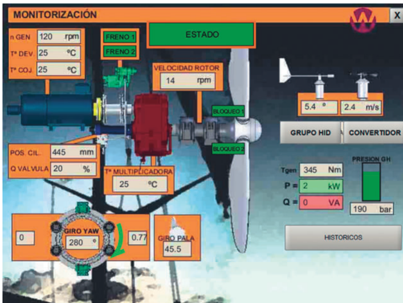
Figura 5. Pantalla de software de monitorización remoto del aerogenerador de 200 kW, modelo Garbí 200/28. Fuente: Electrica Wind, S.L.
