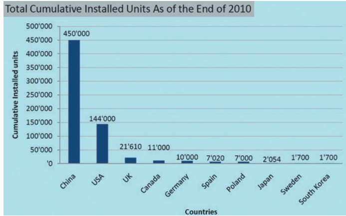
Figura 1.3. Unidades Instaladas en el mundo. Fuente: Small Wind Report 2012 (WWEA).
