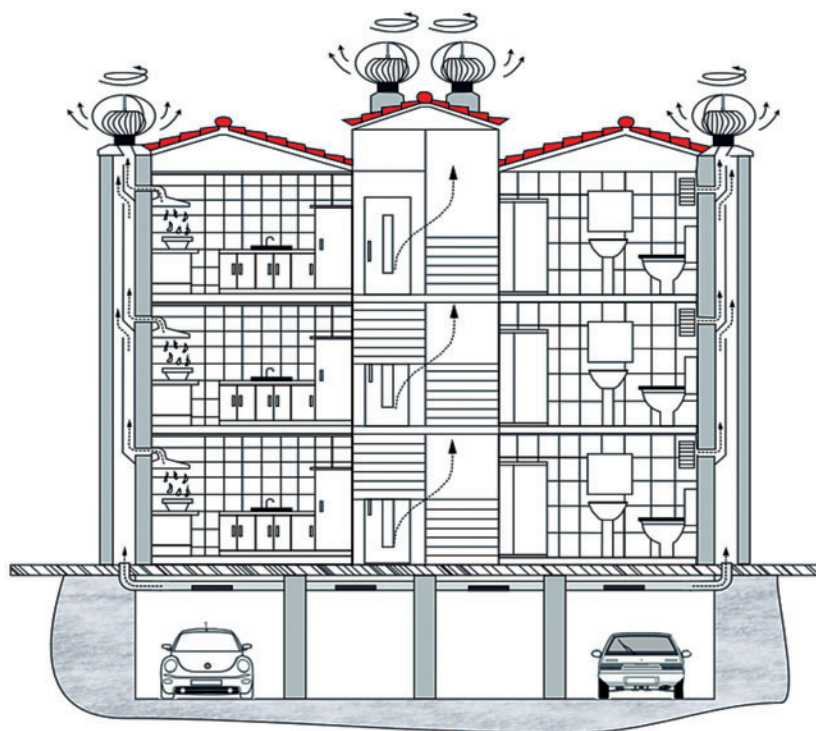
Figura 7. Ilustración acerca de un ejemplo de instalación y funcionamiento en un edificio de viviendas.
