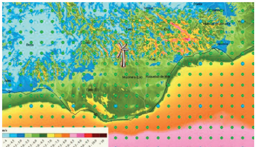
Figura 3. Mapa Eólico a 30m de altura del emplazamiento. Fuente: Electricia.
