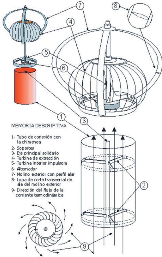
Figura 2. Esquema con las distintas partes del dispositivo. Fuente: Ilustración realizada por F.J. España Moscoso
