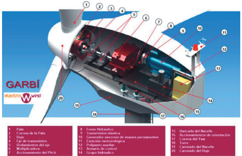
Figura 3. Componentes principales de un aerogenerador de 200 kW, modelo Garbí 200/28. Fuente: Electria Wind, S.L.
