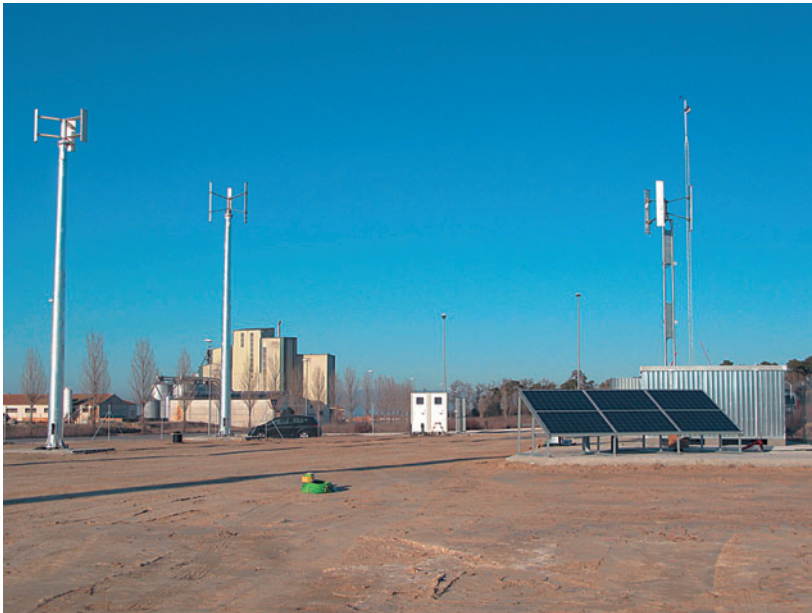
Figura 3. Aerogenerador Technowind. Fuente: CIEMAT.
