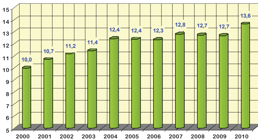
Intensidad gasística (tep/M€ 2002 )
