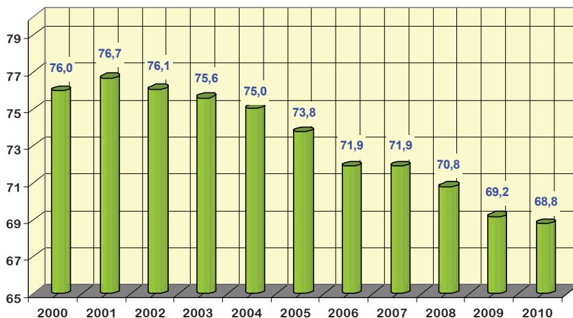
Intensidad energética (tep/M€ 2002 )
