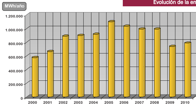
Evolución de la energía eléctrica neta generada
