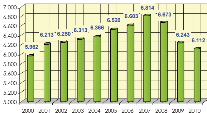
Consumos finales de derivados del petróleo
