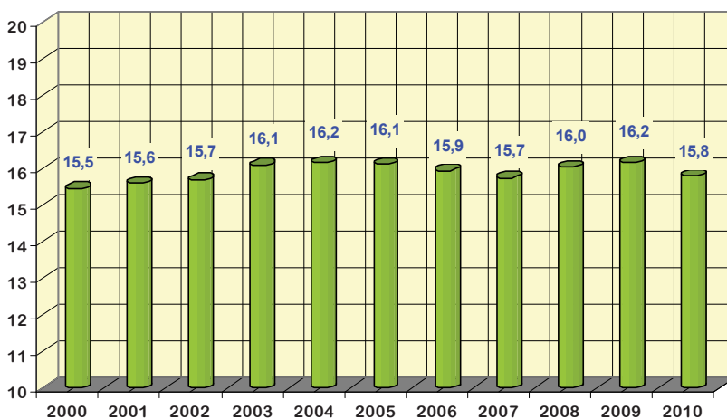
Intensidad eléctrica (tep/M€ 2002 )
