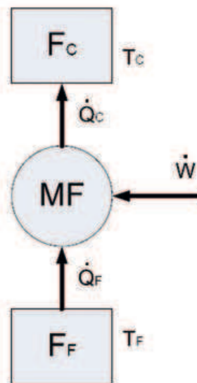
Figura 4. Esquema de principio de máquina frigorífica.
