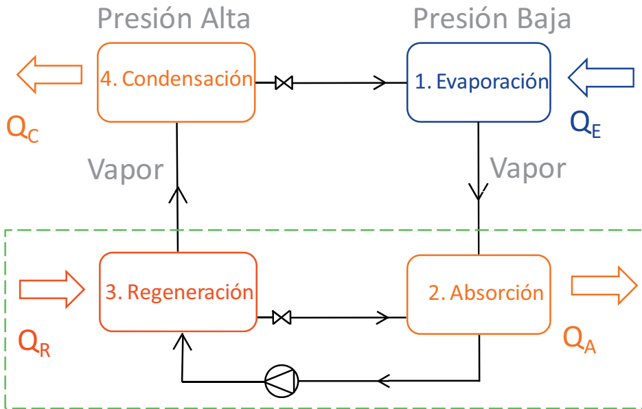
Figura 3. Ciclo de absorción.
