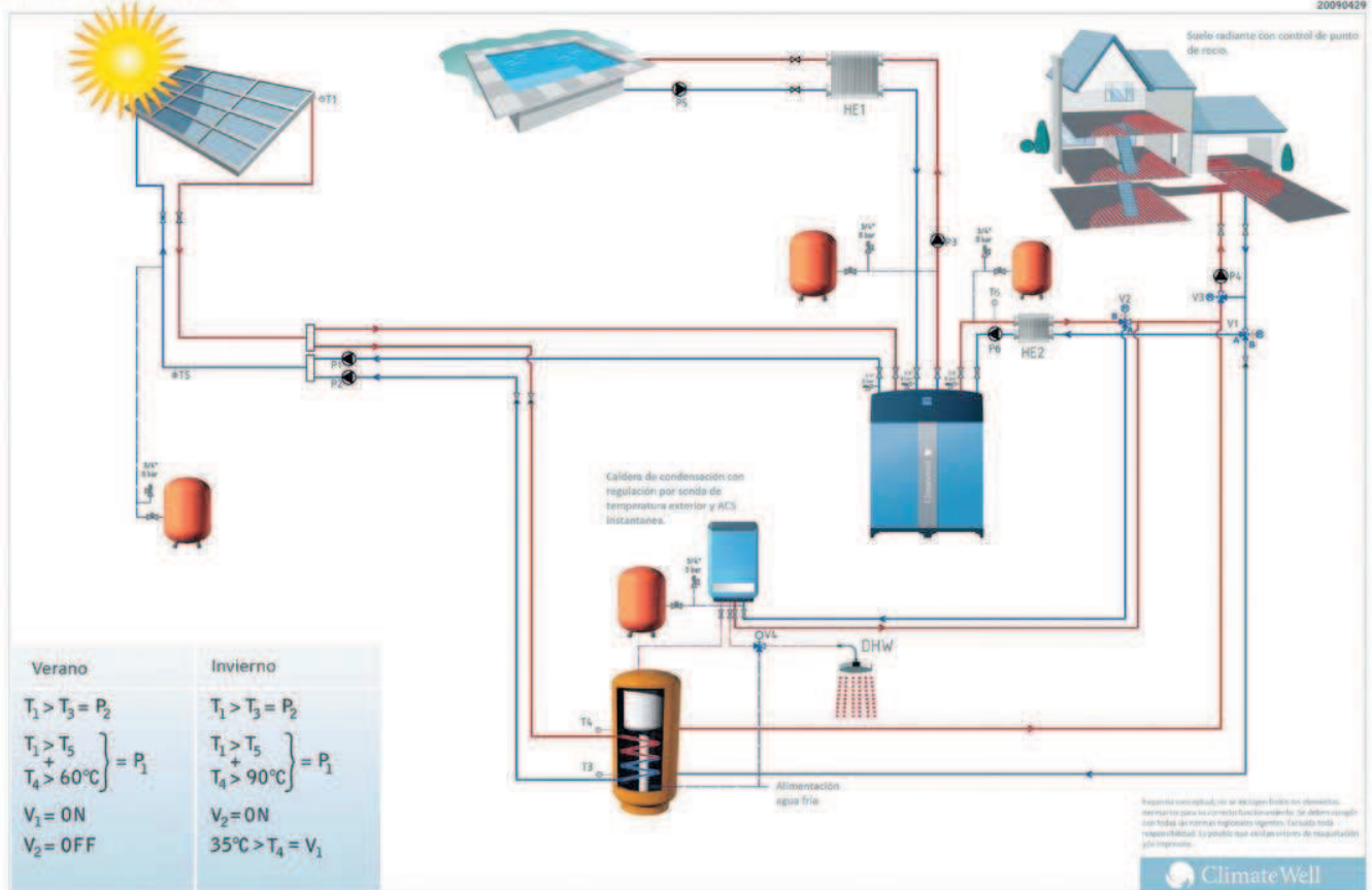
Sistema solar recomendado por ClimateWell Unifamiliar 2 (Sur de España)
