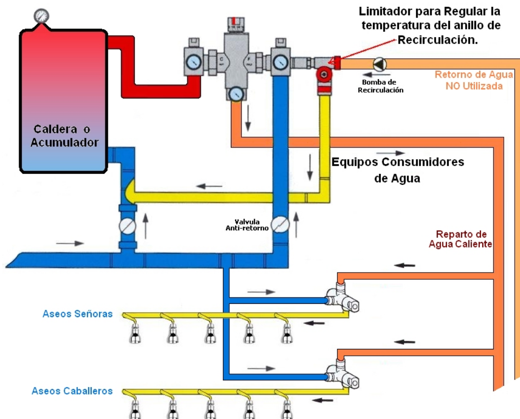
Figura 5. Circuito optimizado de termostatización del agua caliente con anillo de recirculación.
