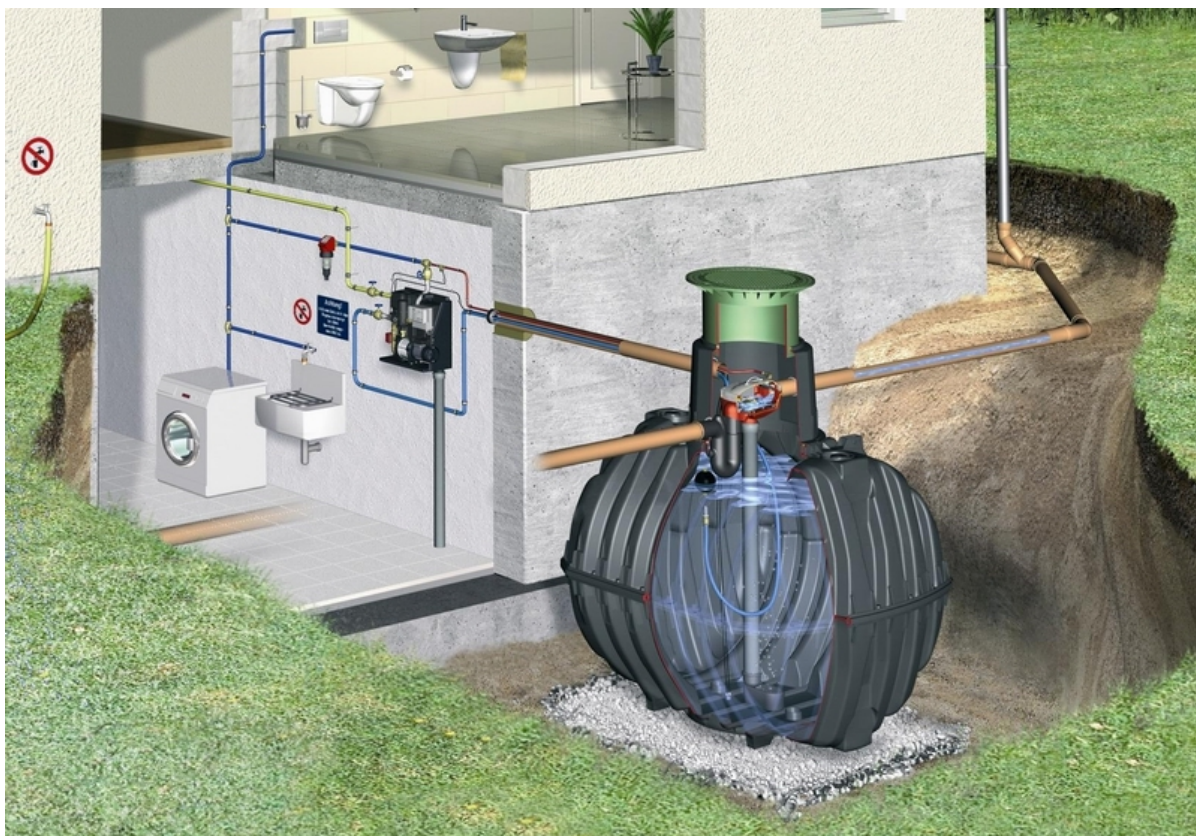
Figura 8. Ejemplo de colector, filtro, depósito y sistema de bombeo de aguas de lluvia.
