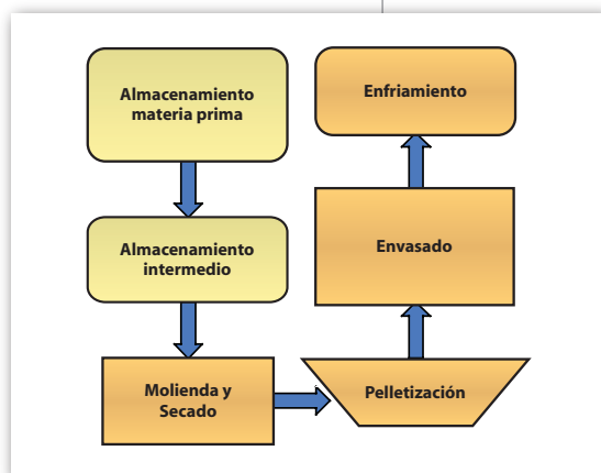
Figura 18: Proceso de pelletización.
