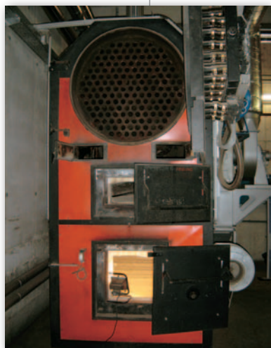
Figura 6: Interior de caldera de parrilla (1.500 kW).
