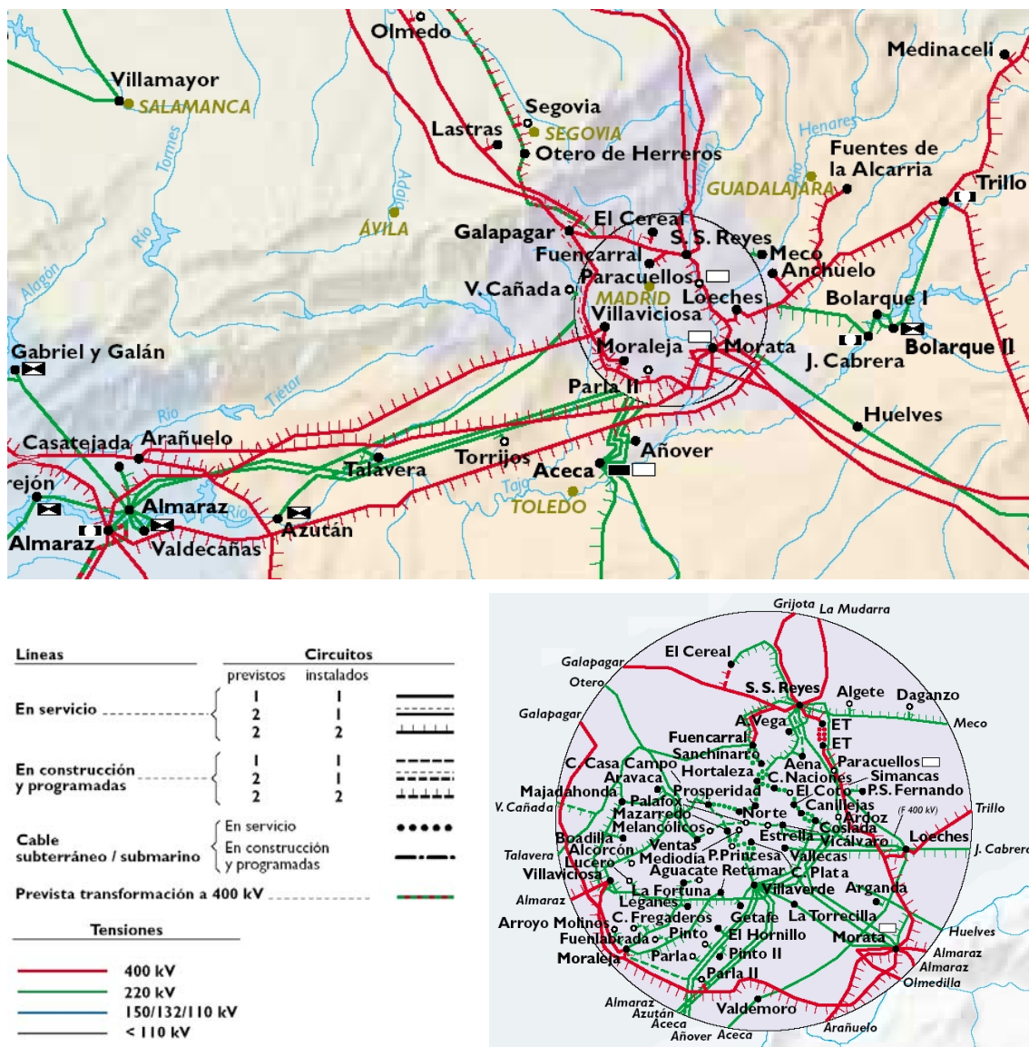
Figura 14. Mapa de la red de transporte de la Comunidad de Madrid y líneas principales de acometida (Fuente: REE).
